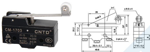
CM-1703
