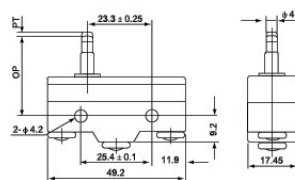
CSSM-25(30)
