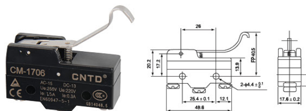
CM-1706
