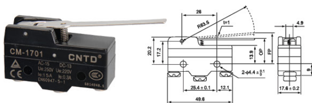
CM-1701
