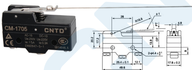
CM-1705
