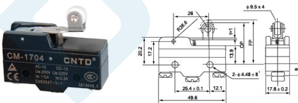
CM-1704
